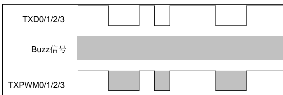
图 4-5 Buzz 低电平调制输出波形图
