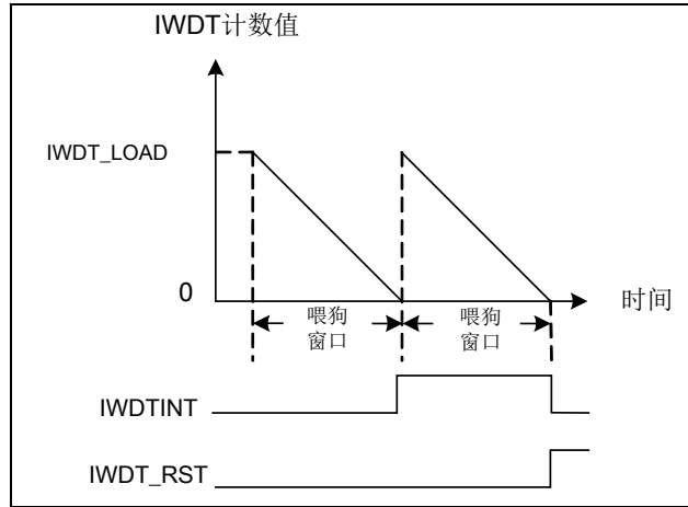
图 5-50 看门狗时序图
