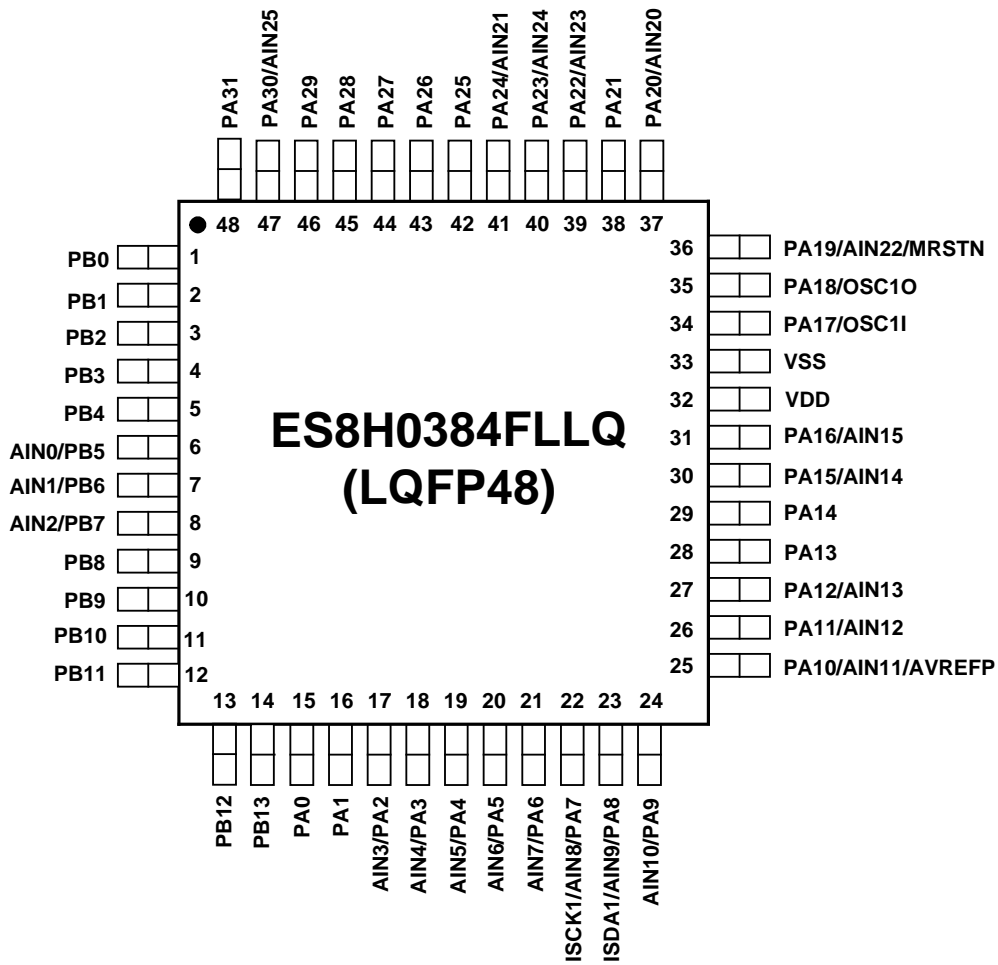
图 1-3 ES8H0384FLLQ LQFP48 封装顶视图
