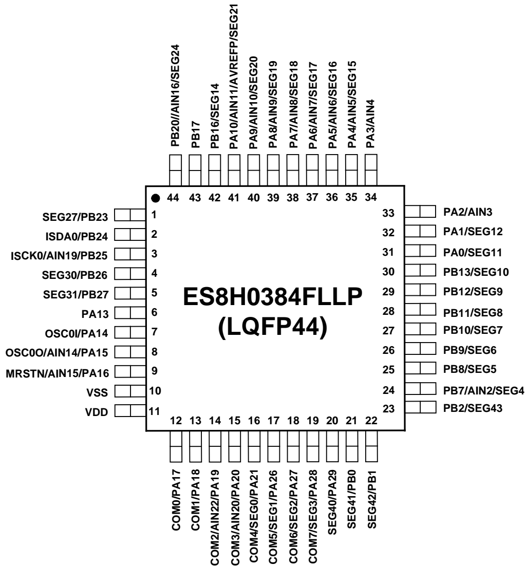
图 1-4 ES8H0384FLLP LQFP44 封装顶视图
