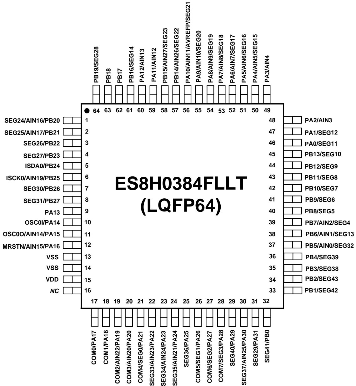
图 1-2 ES8H0384FLLT LQFP64 封装顶视图
