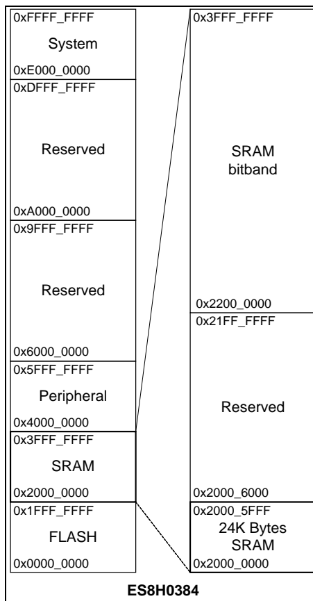
图 3-3 SRAM 映射图
