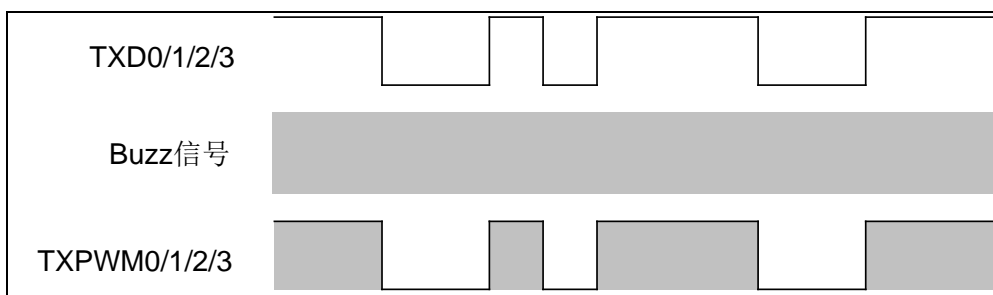
图 4-4 Buzz 高电平调制输出波形图
