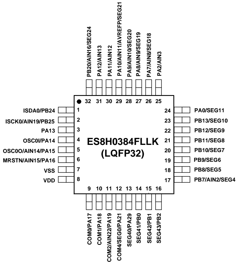
图 1-5 ES8H0384FLLK LQFP32 封装顶视图
